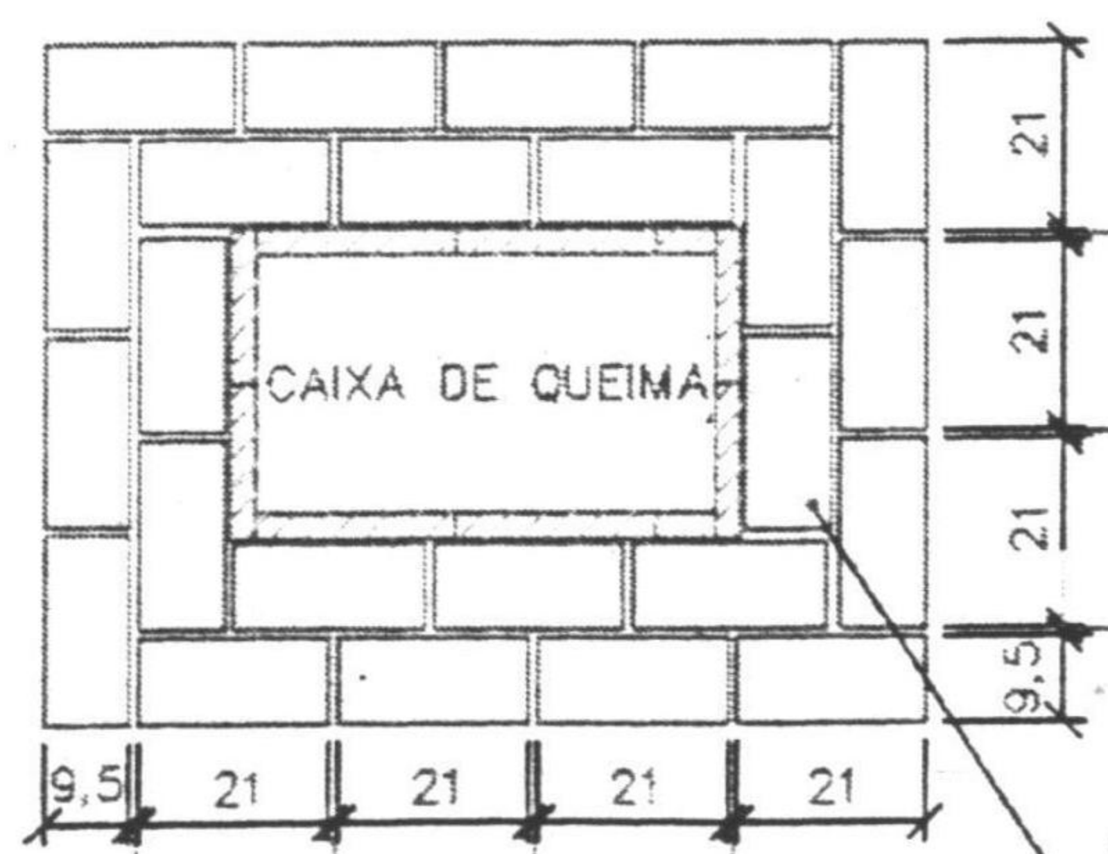
TIPO 1 - PLANTA UTILIZAR TIJOLOS 21x9,5x5
